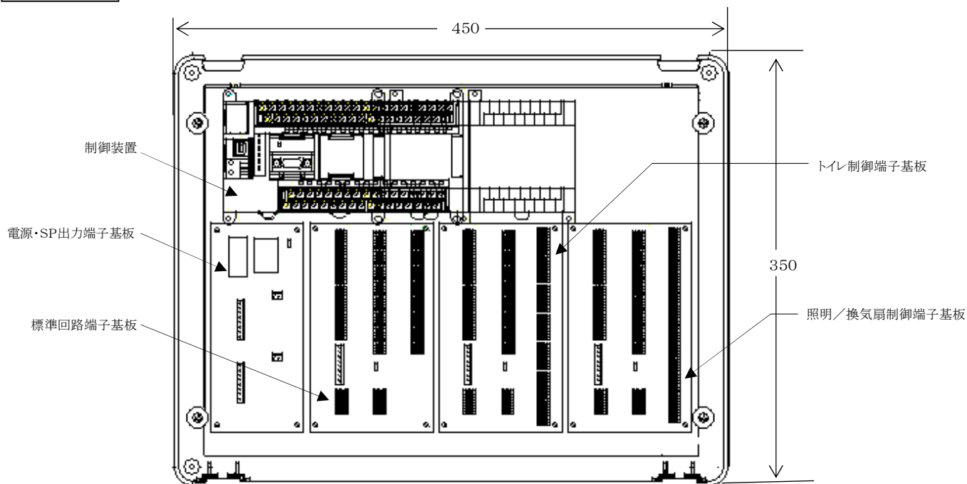
CC24-G-48タイプ装置
